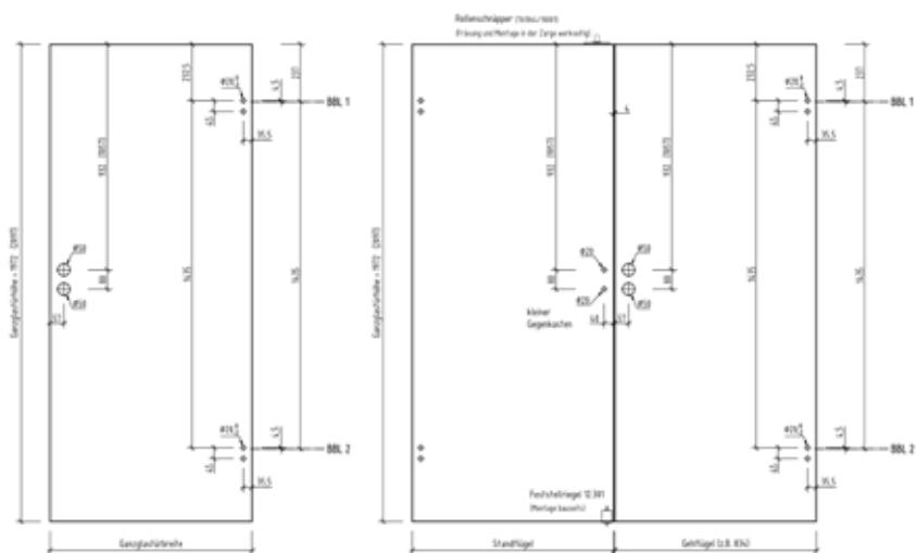
Bohrungsvariante 2 / 1-flg. und 2-flg.
