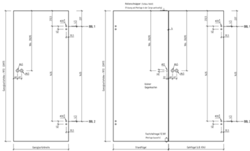
Bohrungsvariante 1 / 1-flg. und 2-flg.
