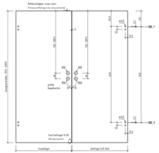
Bohrungsvariante 6, 2-flg.
