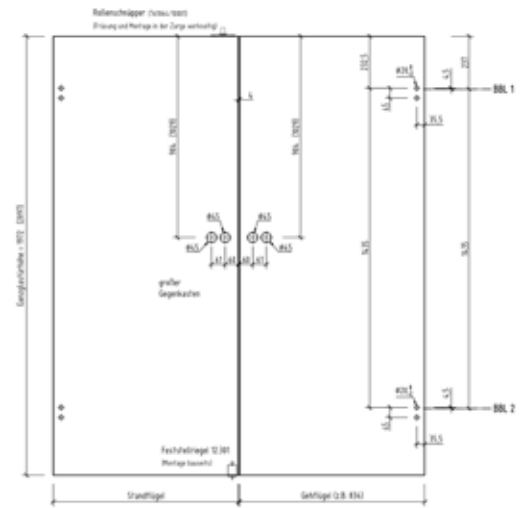
Bohrungsvariante 5, 2-flg.
