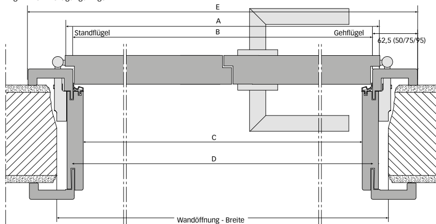
2-flg. Einzelanfertigungszarge
